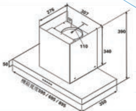
規格圖(單位mm)
